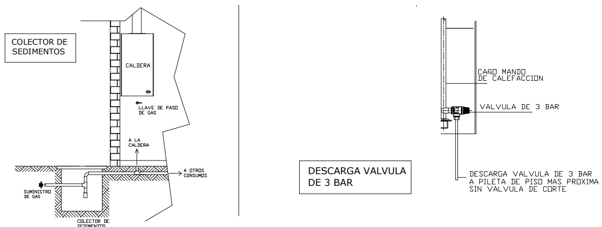
Figura II k: Colector de sedimentos y descarga de Valvula de 3 bar
