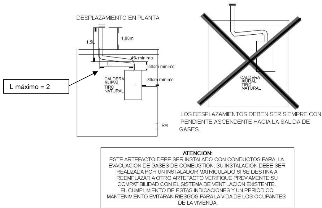
Figura IIg – 1 Salidas de Humo en Tiro Natural
